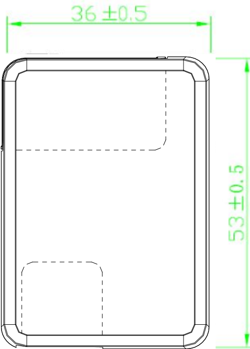
仰视图
